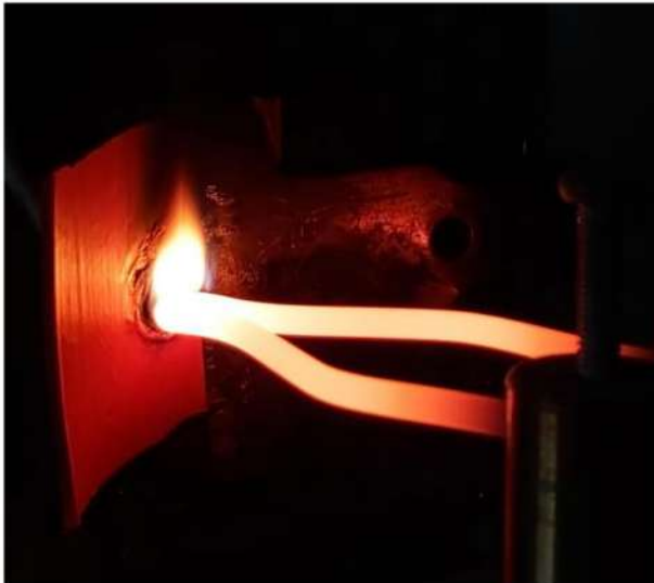
Kızaran Tel Deneyi (Md. 9.1)
