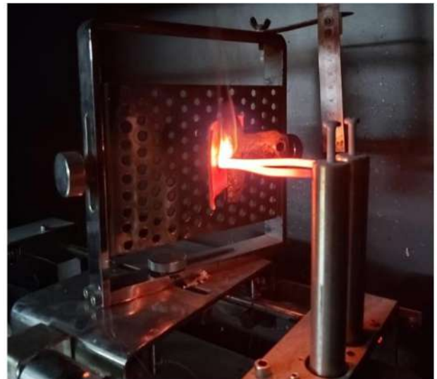
Kızaran Tel Deneyi (Md. 9.1)
